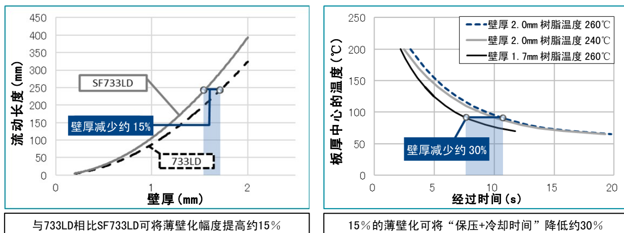
图2-2 高流动性与薄壁化
