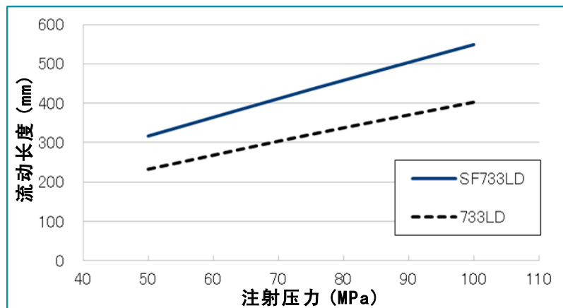
图3-1 棒流动长度 (2mmt)
