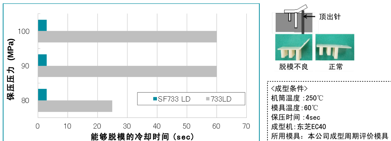
图2-1 SF733LD与733LD的脱模性比较
